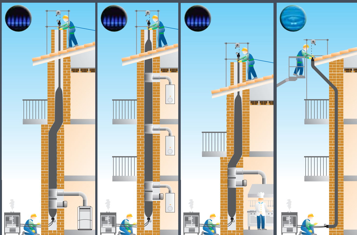
Esempi di installazione della manichetta FuranFlex®
